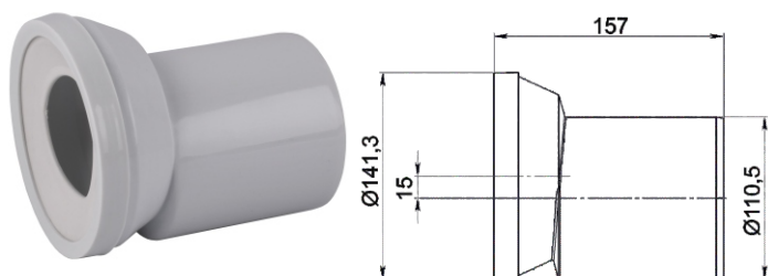
Патрубок для унітазу зі зміщенням 15 мм Арт.: OPTI 51110/155 Діаметр: 110 мм Довжина: 155 мм Матеріал: пластик, гума Код: 31824
