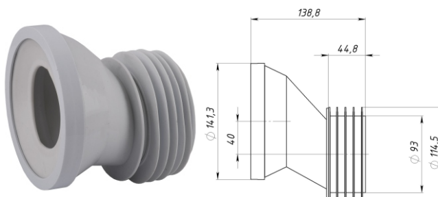
Патрубок для унітазу зі зміщенням 20 мм та ущільненням Арт.: OPTI 60115/120 Діаметр: 115 мм Довжина: 120 мм Матеріал: пластик, гума Код: 31821
