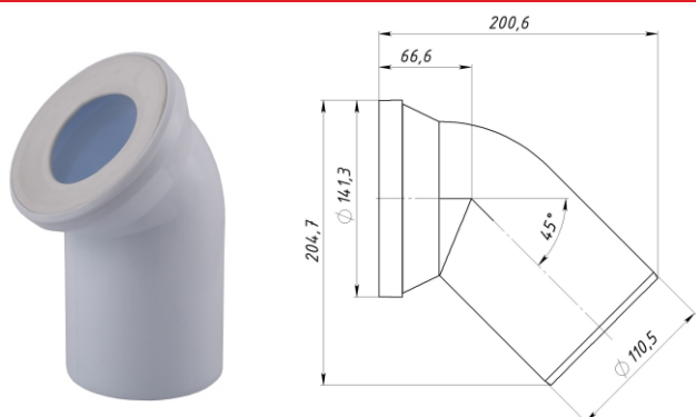
Коліно для унітазу Арт.: OPTI 31410/227 Кут нахилу: 45° Діаметр: 110 мм Матеріал: пластик, гума Код: 31819
