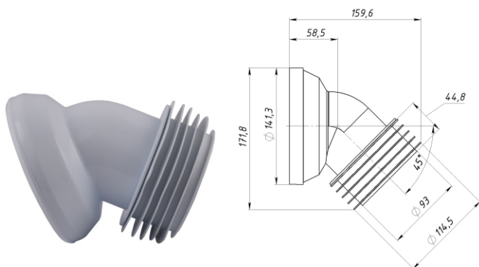
Коліно для унітазу Арт.: OPTI 30515/147 Кут нахилу: 45° Діаметр: 115 мм Матеріал: пластик, гума Код: 31823
