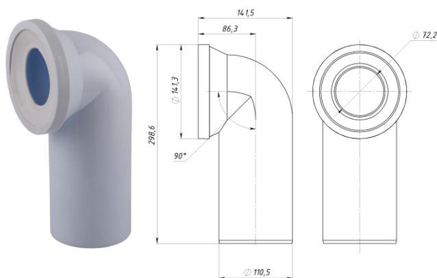
Коліно для унітазу Арт.: OPTI 41410/296 Кут нахилу: 90° Діаметр: 110 мм Матеріал: пластик, гума Код: 31820
